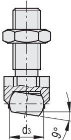
GN 709.3-B
